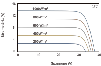
Strom-Spannungs- und Leistungs-Spannungs-Kurve (440)
