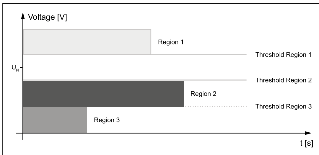
Einteilung des Netzspannungsbereichs in 3 Störungsregionen durch Wahl der Erkennungsschwellen.
