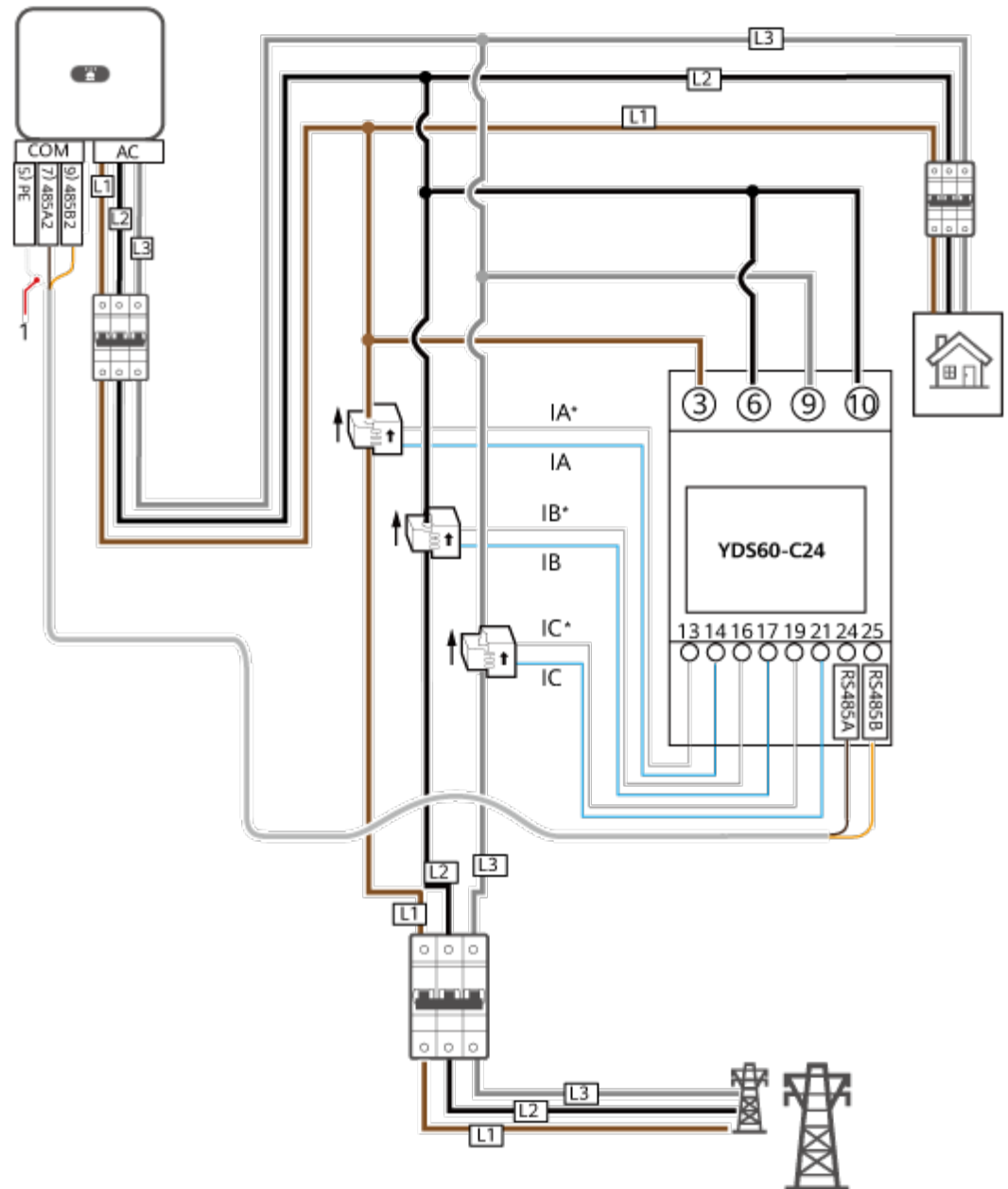
Abbildung 5-28 Dreiphasige, dreiadrige Kabelverbindung mit YDS60-C24 (Smart Dongle-Vernetzung)
