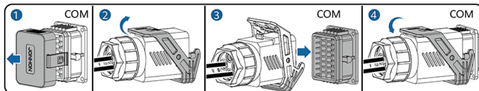
Abbildung 5-26 Sichern des Signalkabelanschlusses
