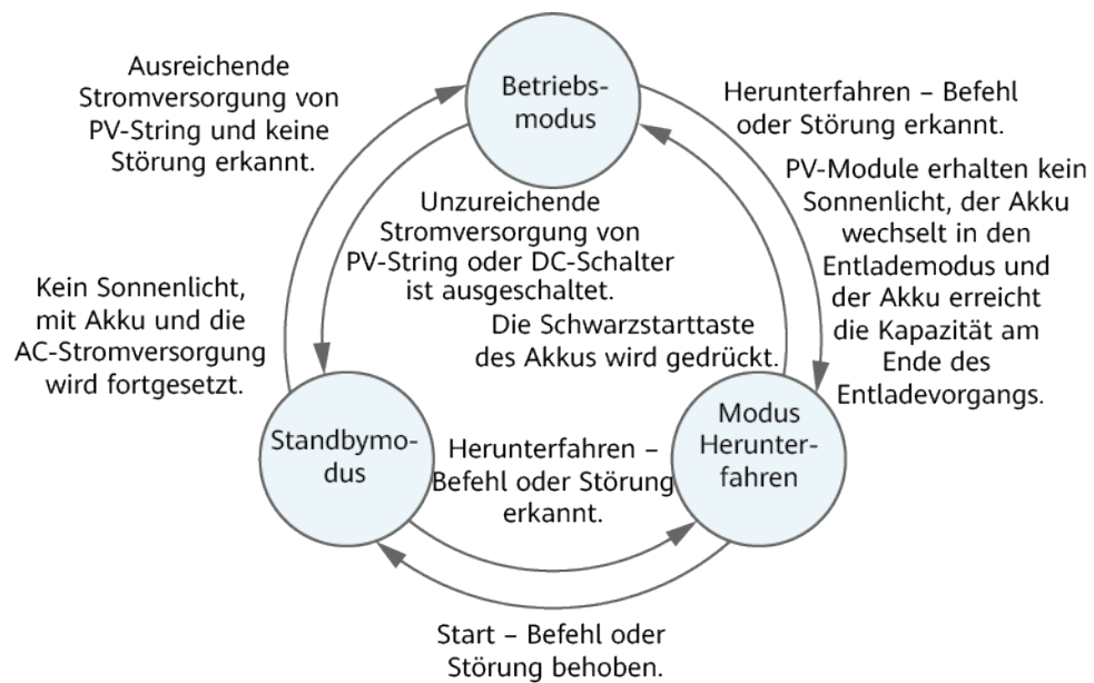
Abbildung 2-6 Arbeitsmodi
