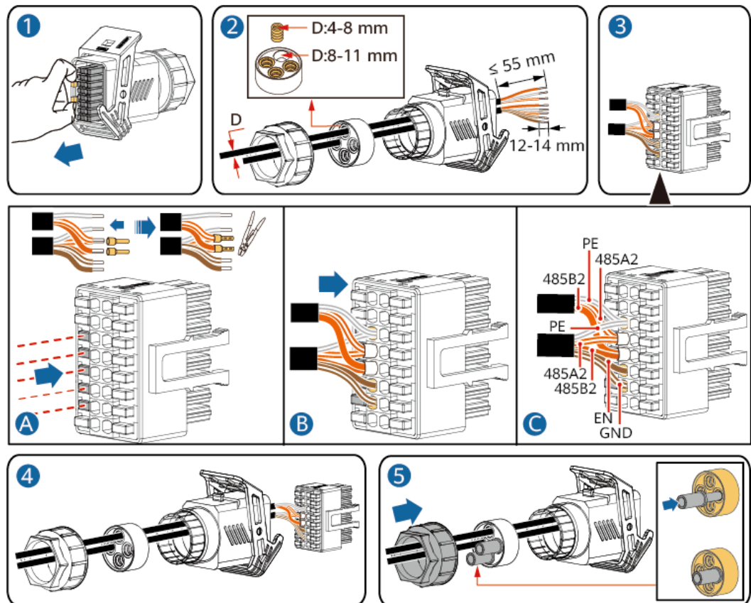
Abbildung 5-32 Kabelmontage
