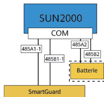
Abbildung 5-24 SmartGuard-Vernetzung (die Komponente im gestrichelten Kasten ist optional)
