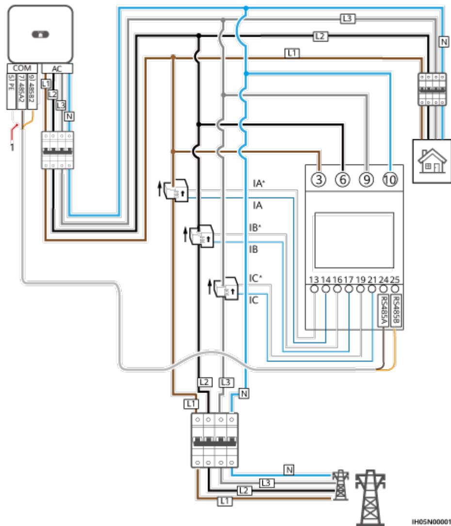
Abbildung 5-29 Dreiphasige vieradrige Verbindung (Smart Dongle-Netzwerk)
