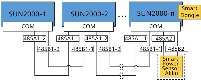
Abbildung 5-21 Smart Dongle-Netzwerkaufbau (gestrichelte Linie kennzeichnet optionale Komponenten)
