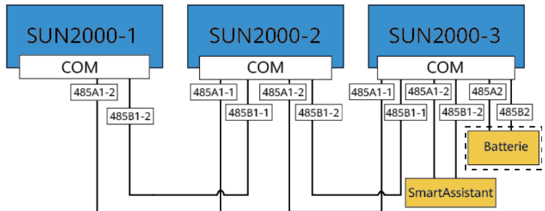
Abbildung 5-23 SmartAssistant-Vernetzung (die Komponente im gestrichelten Kasten ist optional)
