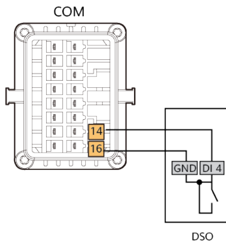
Abbildung 7-5 Kabelverbindungen
