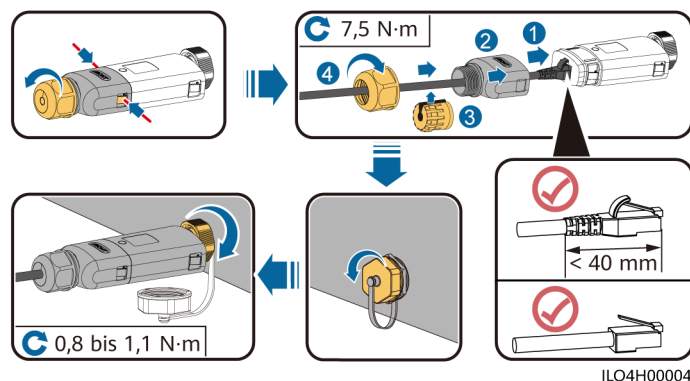
Abbildung 5-16 Installieren von WLAN-FE-Smart Dongle (FE-Kommunikation)
