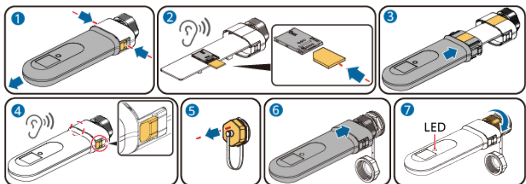
Abbildung 5-18 Installieren von 4G Smart Dongle (SDongleB-06)
