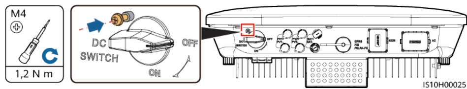
Abbildung 4-16 Montieren der Sicherungsschraube für den DC-Schalter
