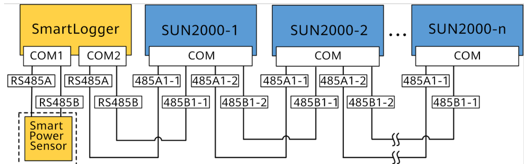
Abbildung 5-22 SmartLogger-Netzwerkaufbau (gestrichelte Linie kennzeichnet optionale Komponenten)
