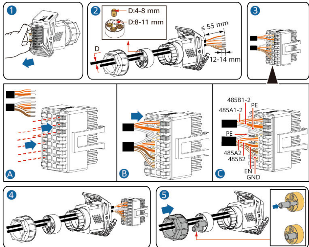
Abbildung 5-36 Installieren von Kabeln
