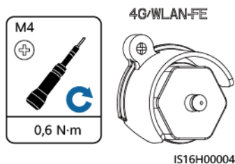
Abbildung 5-19 Installation der Anti-Diebstahl-Komponenten für den Smart Dongle
