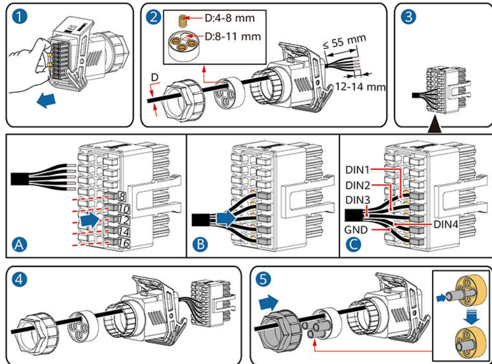
Abbildung 5-42 Kabelmontage
