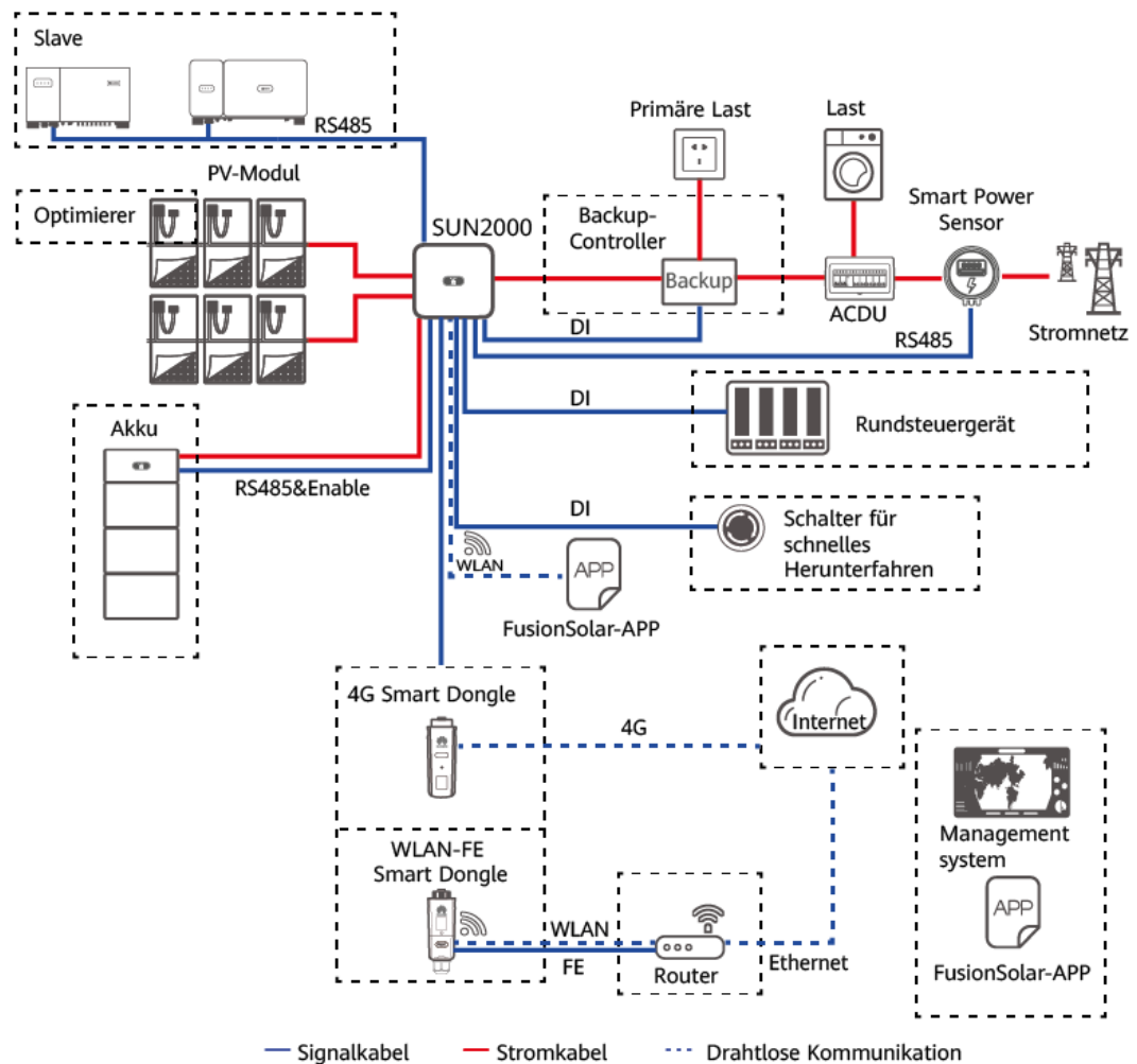
Abbildung 2-2 Netzanwendung (gestrichelte Linien kennzeichnen optionale Komponenten)
