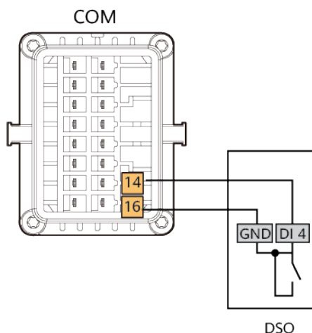
Abbildung 7-10 Kabelverbindungen
