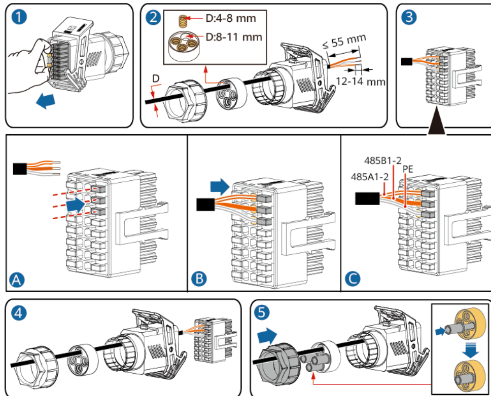
Abbildung 5-34 Kabelmontage
