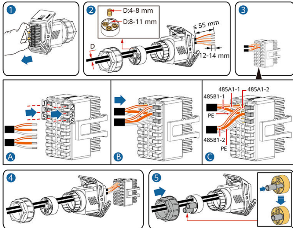
Abbildung 5-25 Kabelmontage
