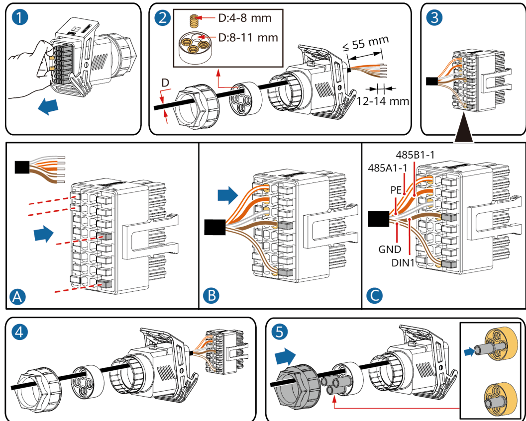
Abbildung 5-38 Kabelmontage
