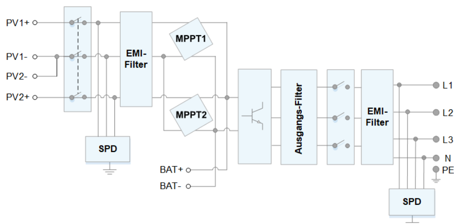
Abbildung 2-5 Konzeptdiagramm des SUN2000
