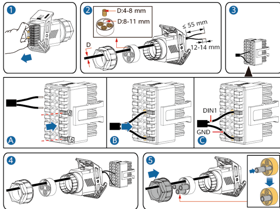
Abbildung 5-44 Kabelmontage
