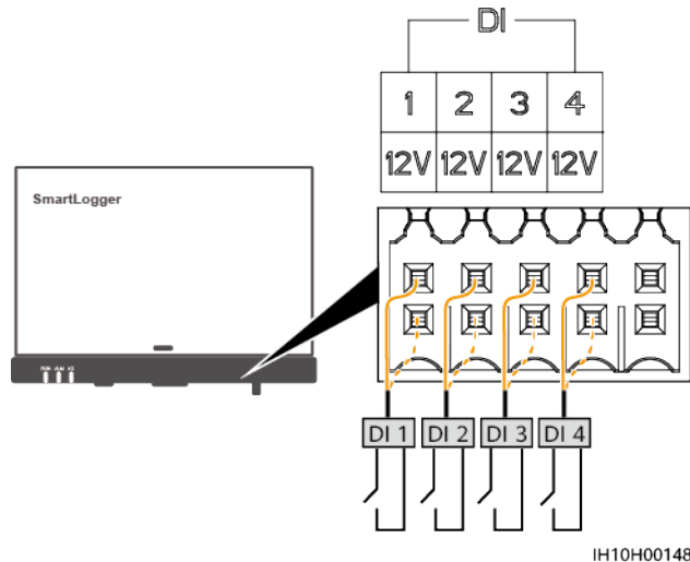
Abbildung 5-41 Kabelverbindungen (SmartLogger-Vernetzung)
