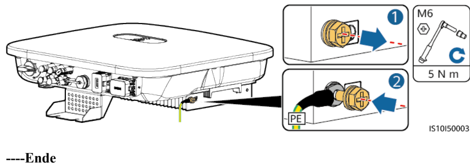
Abbildung 5-3 Anschließen des PE-Kabels
