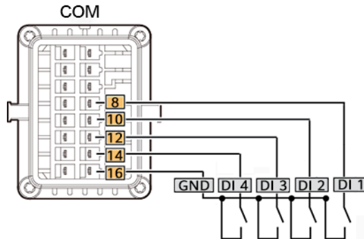
Abbildung 5-40 Kabelverbindungen (Smart Dongle-, SmartAssistant- und SmartGuard-Vernetzung)
