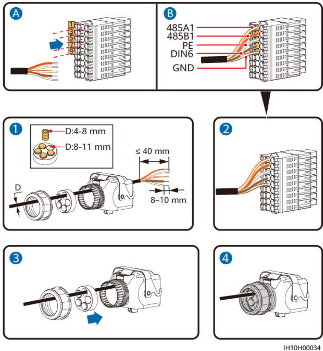
Abbildung 5-30 Kabelmontage
