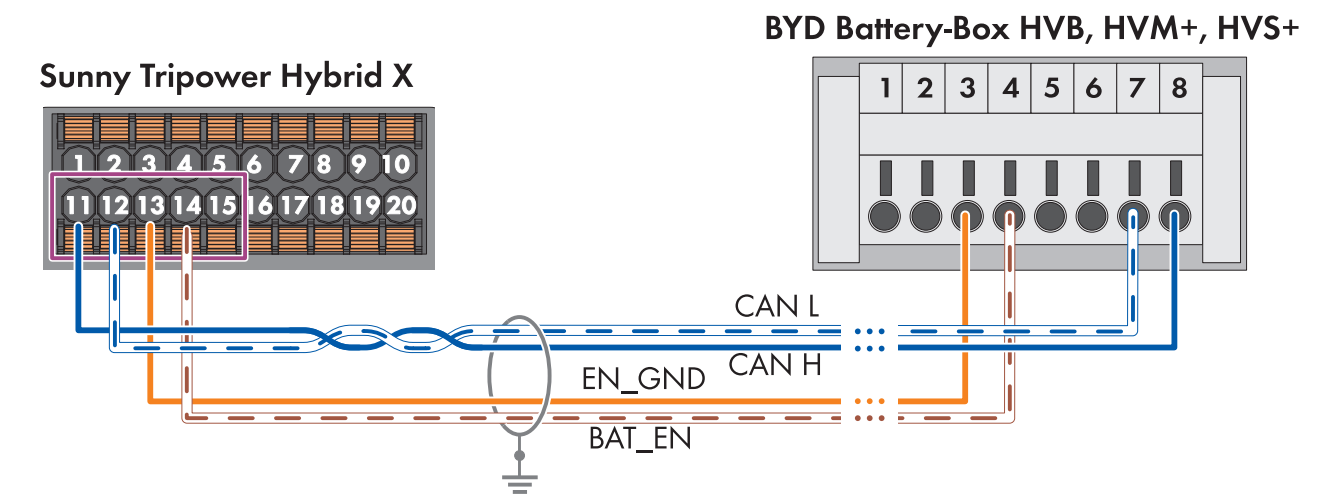
Abbildung 4: Verkabelungsprinzip für die Verschaltung von Sunny Tripower Hybrid X mit BYD Battery-Box HVB, HVM+ und HVS+.
