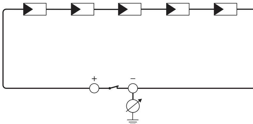
Abbildung 14: Schematische Darstellung der Messung
