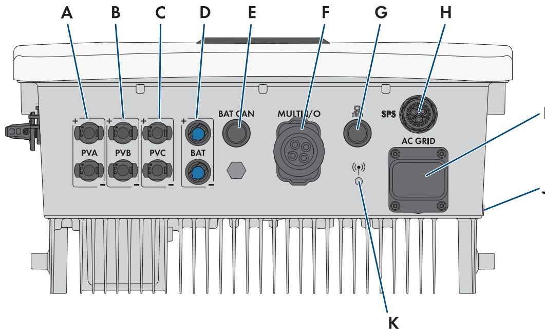
Abbildung 7: Unteransicht des Wechselrichters
