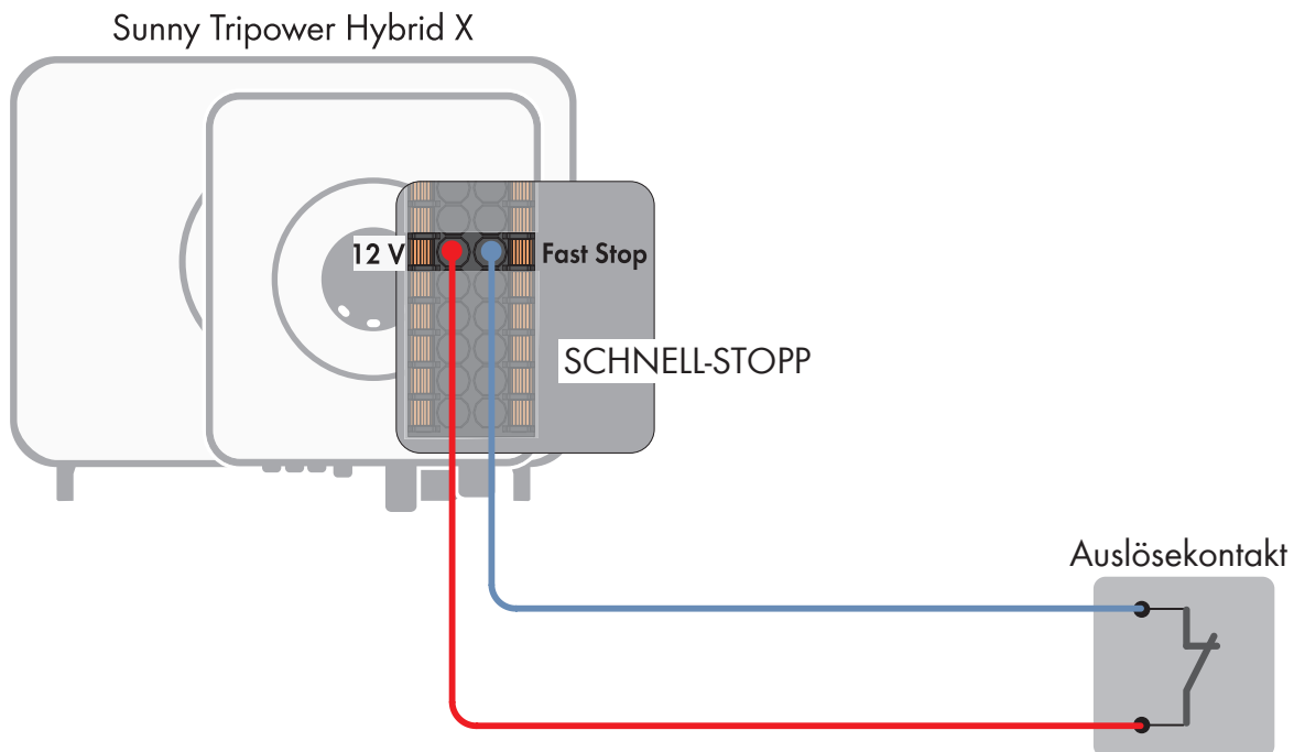
Abbildung 11: Beispiel der Verschaltung für den Anschluss eines Auslösekontakts für den Schnell-Stopp.
